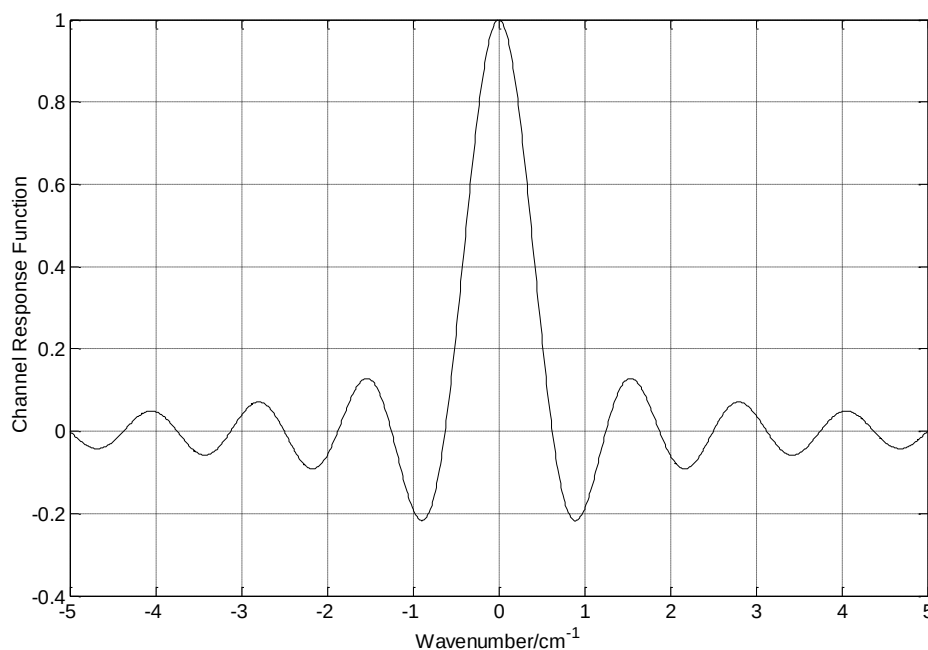
图 4 HIRAS-II Sinc 函数形式的通道光谱响应函数，其峰值半宽 \text{FWHM}=1.21/(2\text{MPD})
